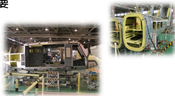
陸自多用途ヘリコプター (UH-1J) における定期機体整備の様子
